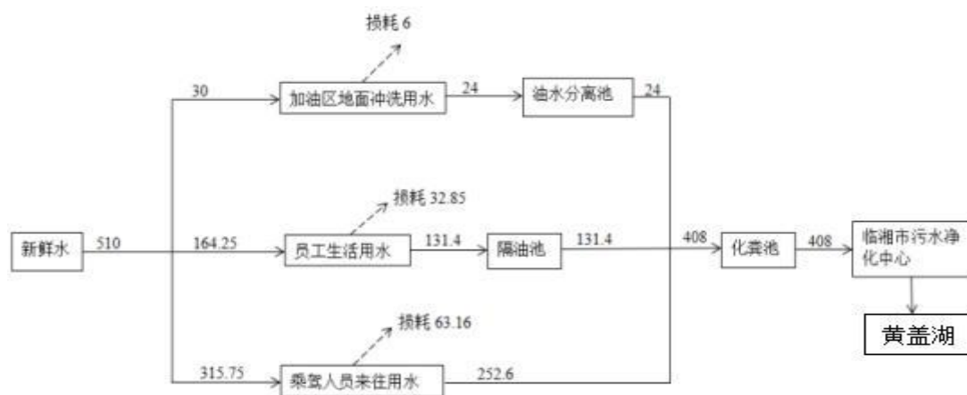
图 3.5-1 项目水平衡图 (单位 m^3/d )
